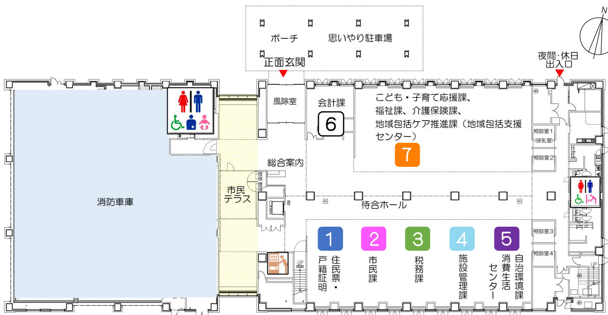
1階平面図
