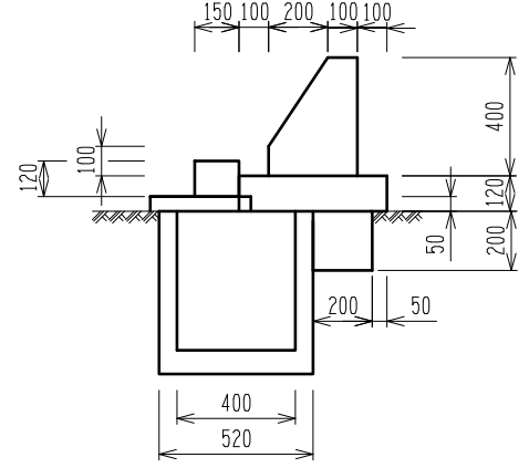
墓誌 正面図
